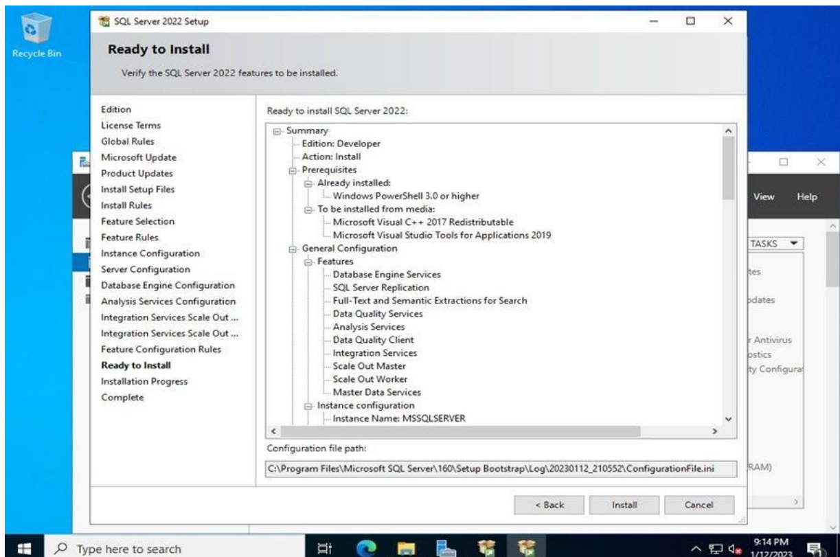
Hình 3.15. Kiểm tra lại tất cả các cấu hình đã chọn
