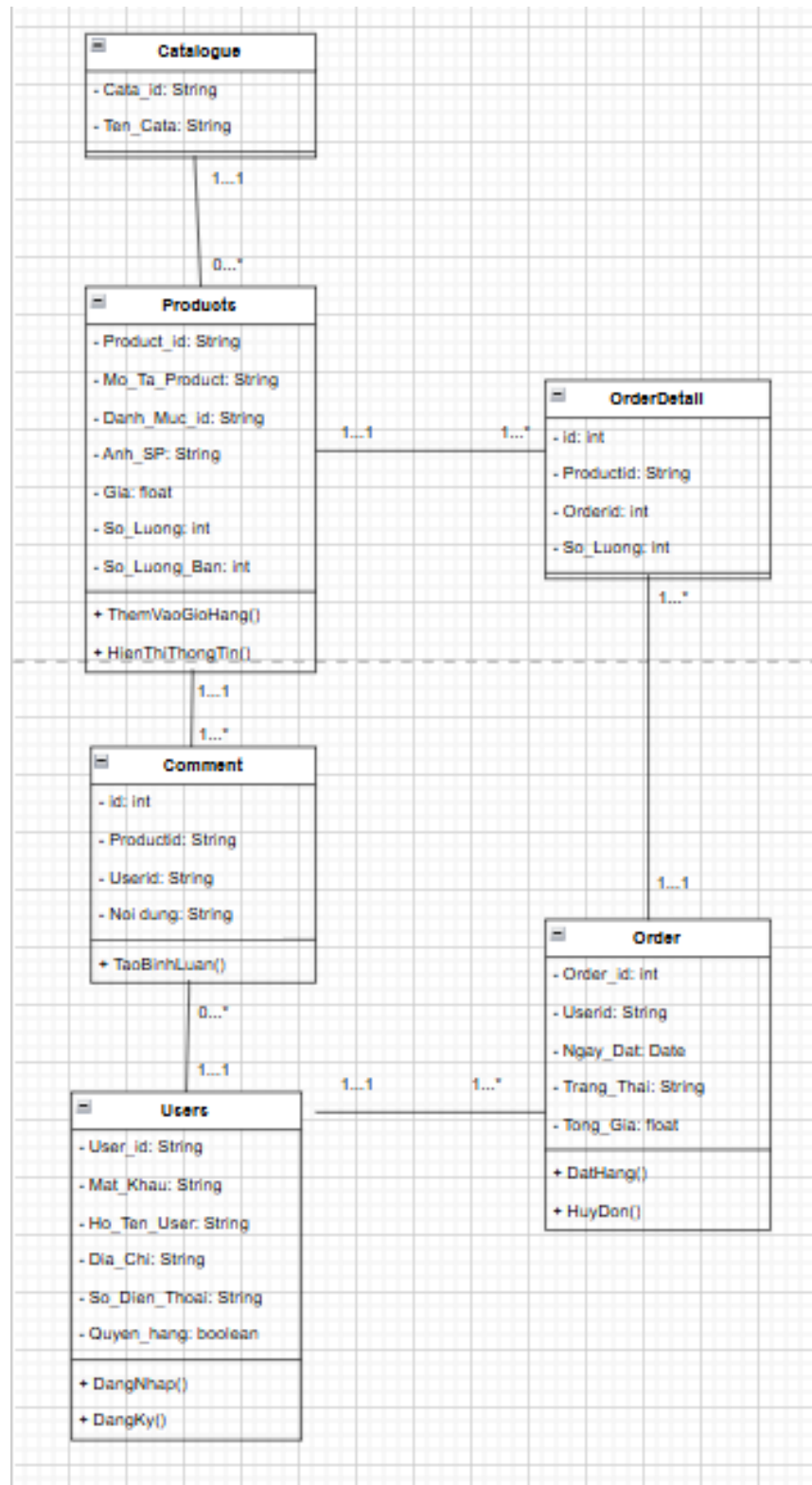
Hình 2.8. Sơ đồ lớp
