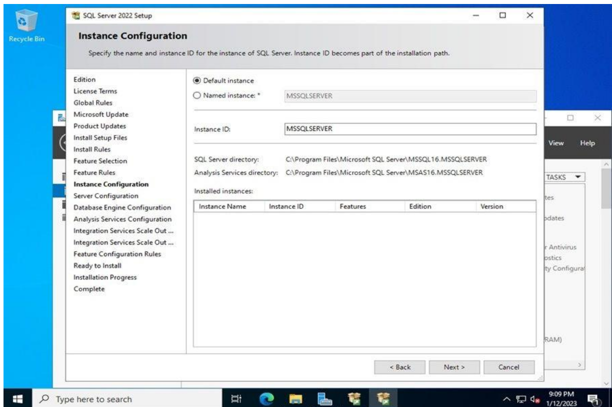
Hình 3.10. Chọn Default instance nếu bạn muốn cài đặt mặc định
