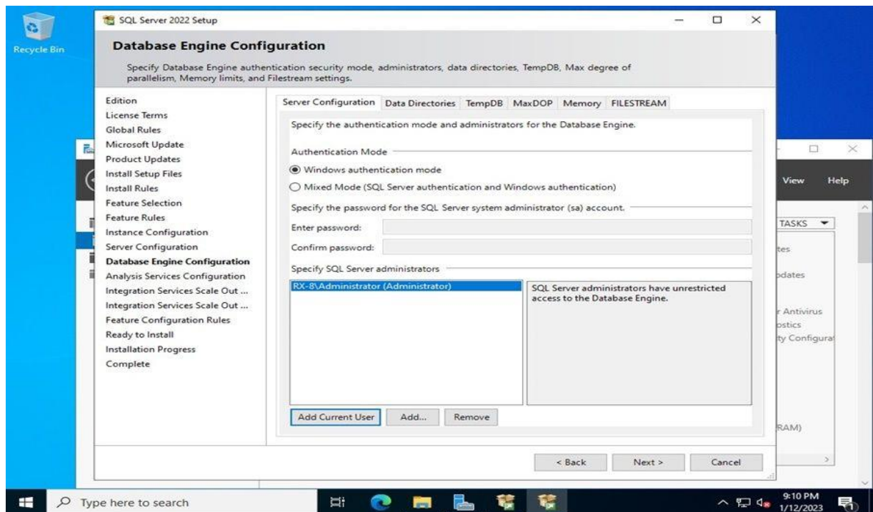
Hình 3.12. Database Engine Configuration
