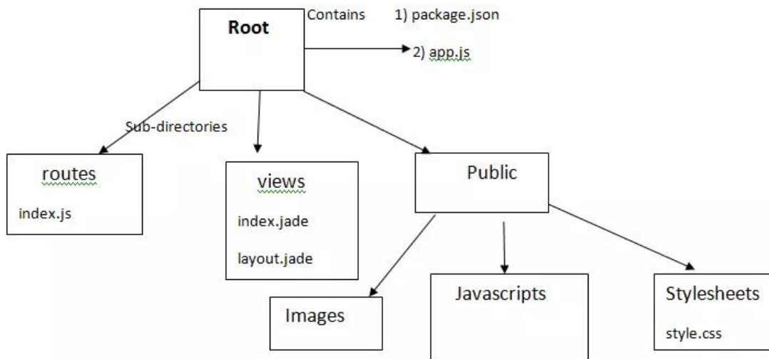
Hình 1.3. Mô hình ExpressJS
