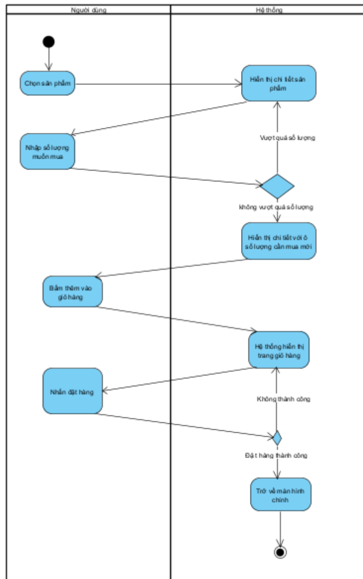
Hình 2.3. Sơ đồ hoạt động đặt hàng
