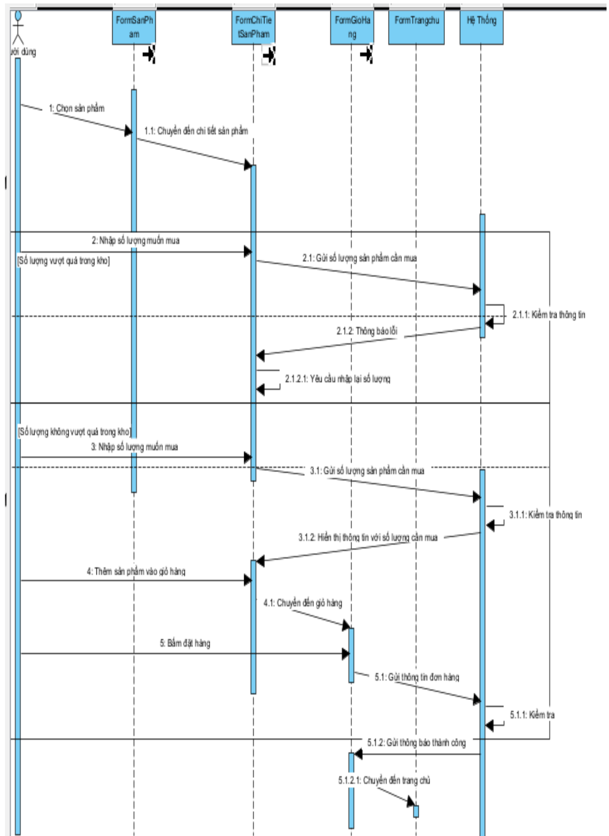
Hình 2.5. Sơ đồ trình tự đặt hàng
