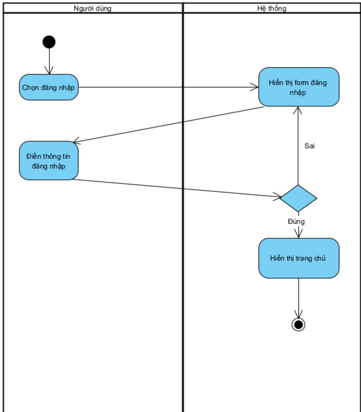
Hình 2.2. Sơ đồ hoạt động đăng nhập
