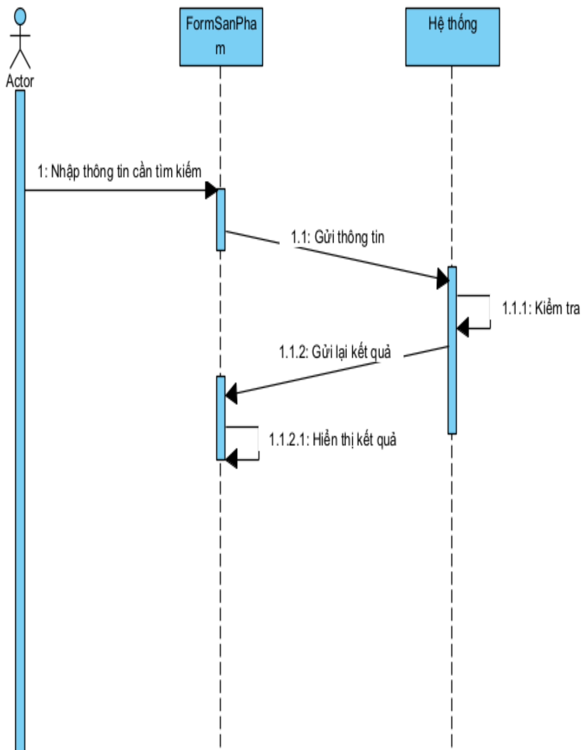
Hình 2.6. Sơ đồ Tuần tự tìm kiếm Sản Phẩm
