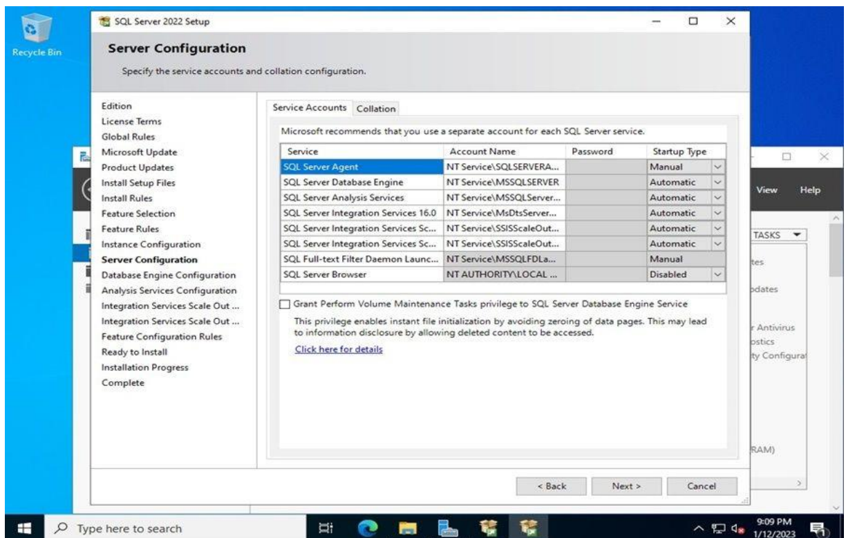
Hình 3.11. Chọn tài khoản người dùng cho các dịch vụ SQL Server
