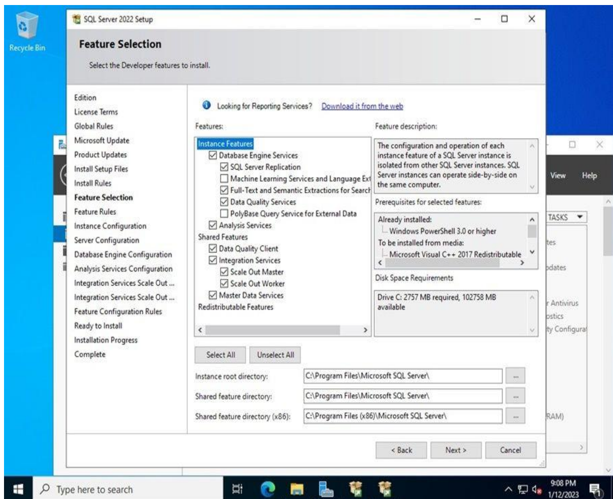
Hình 3.9. Chọn các tính năng mà bản thân muốn cài đặt
