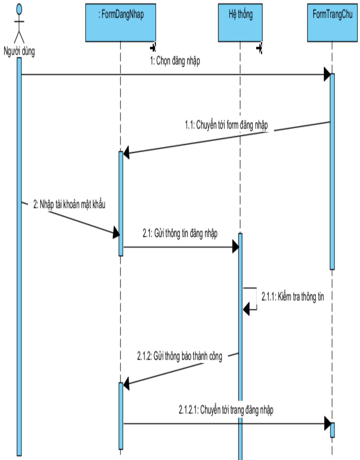
Hình 2.4. Sơ đồ trình tự đăng nhập
