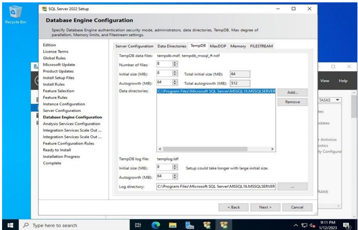
Hình 3.14. Cấu hình TempDB nếu cần điều chỉnh thông số mặc định
